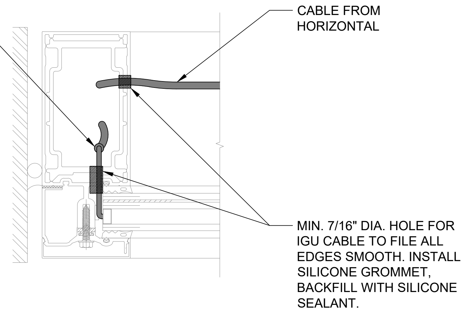
DETAIL 4 LEFT JAMB
